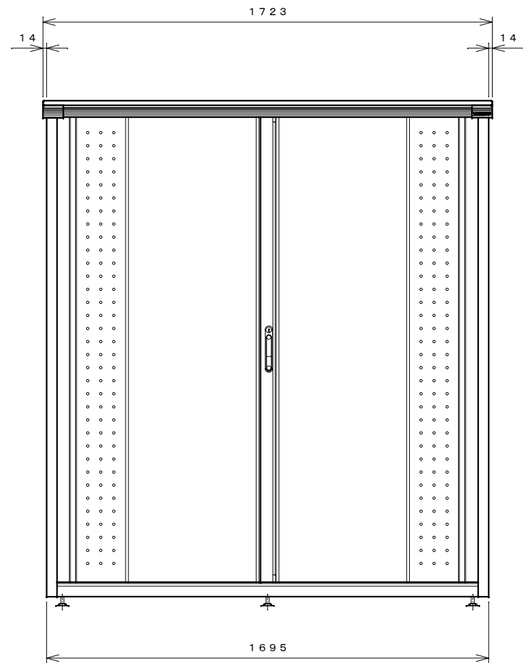
正面図
